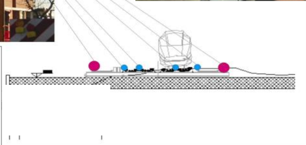
Rappresentazione schematica dell'impianto di monitoraggio ed elaborazione dati
