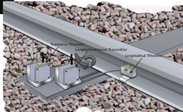
Sensori di inclinazione wireless
